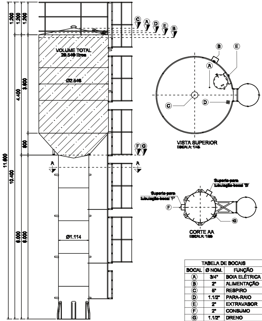
VISTA LATERAL ESCALA: 1/80
